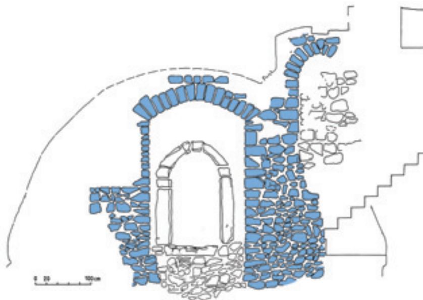
Ściana północna najstarszego budynku z przełomu XIII i XIV w. w tzw. Sali Gotyckiej Collegium Minus, stan obecny; w latach 1428–1475 siedziba Bursy Divitum. Rys. E. Grochowska i D. Niemiec na podstawie wyników badań S. Sławińskiego oraz D. Niemca (relikty najstarszej kamienicy z XIII/XIV w. zaznaczono kolorem niebieskim)
